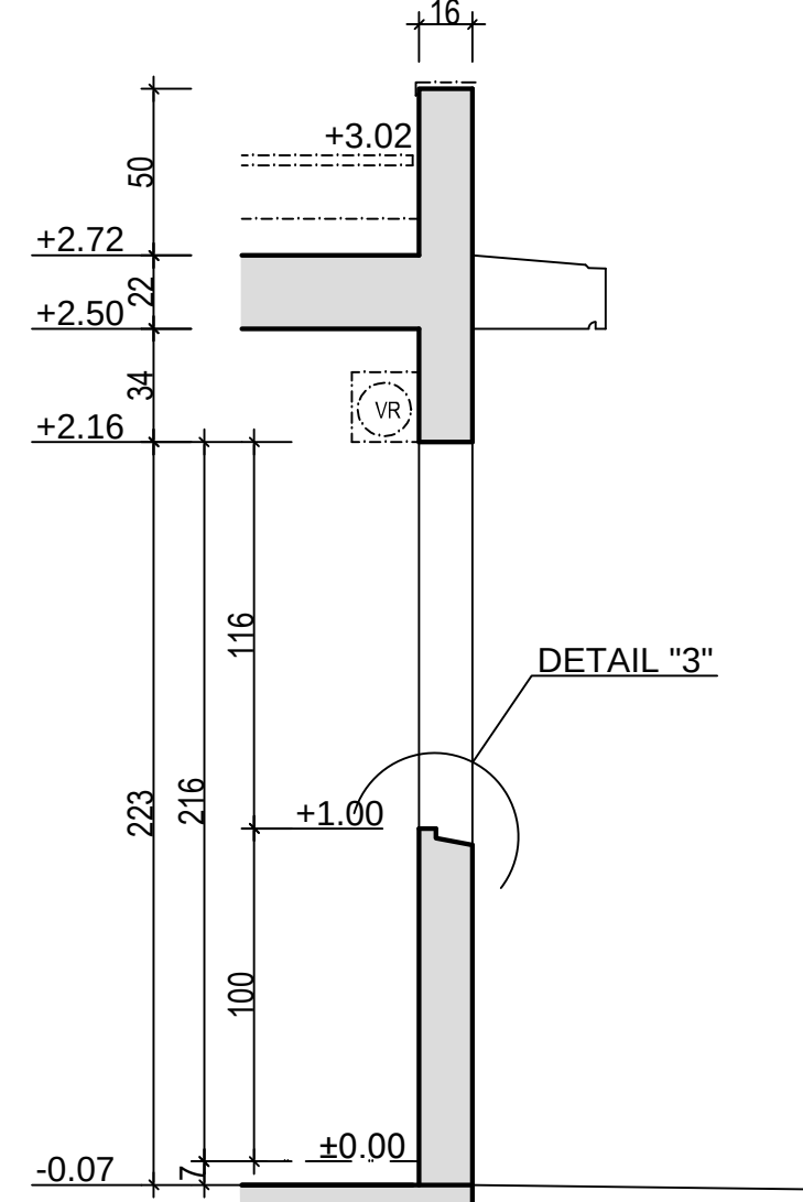
COUPE D Ech: 1/25
