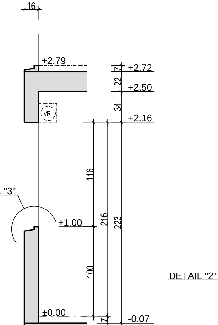
COUPE H Ech: 1/25
