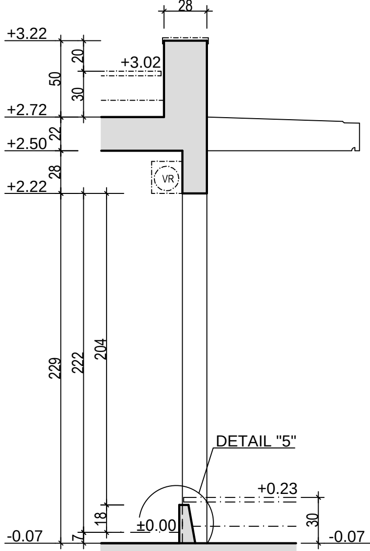
COUPE B Ech: 1/25
