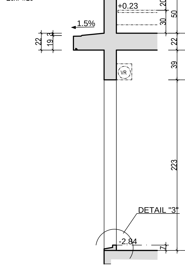
COUPE M Ech: 1/25
