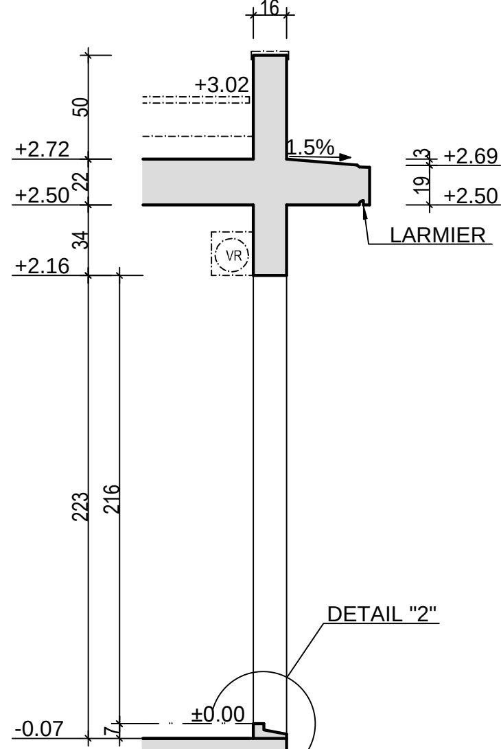
COUPE C Ech: 1/25
