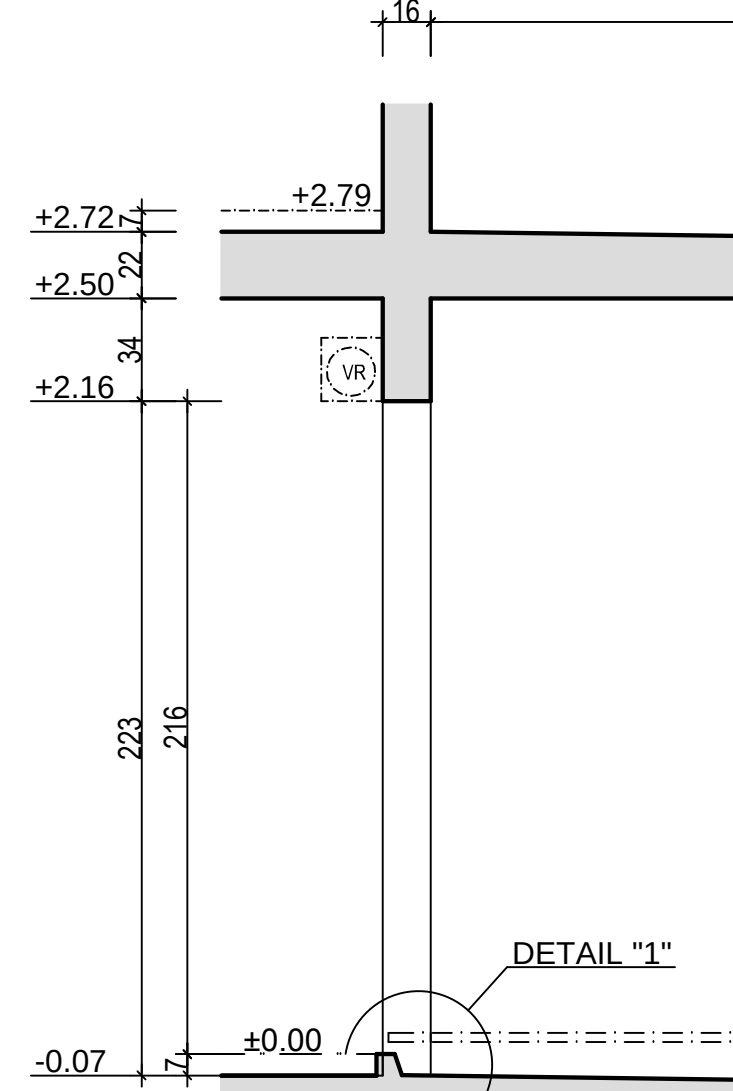
COUPE G Ech: 1/25
