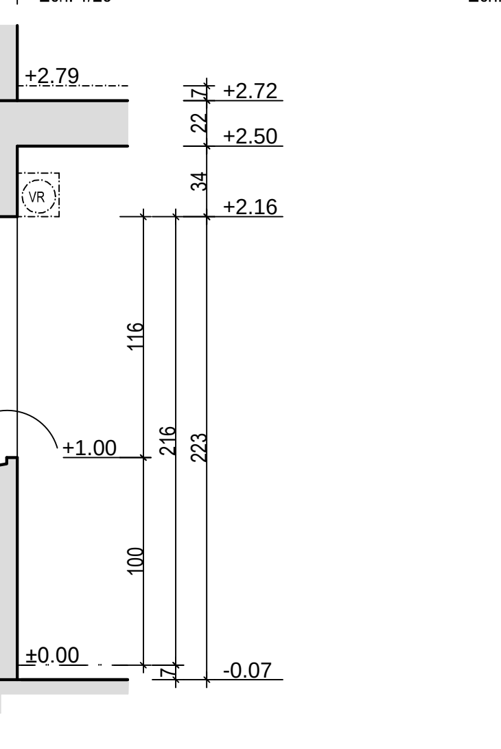
COUPE L Ech: 1/25
