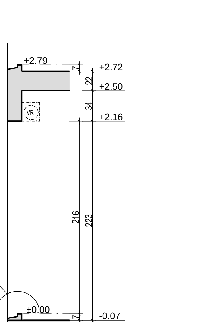
COUPE J Ech: 1/25
