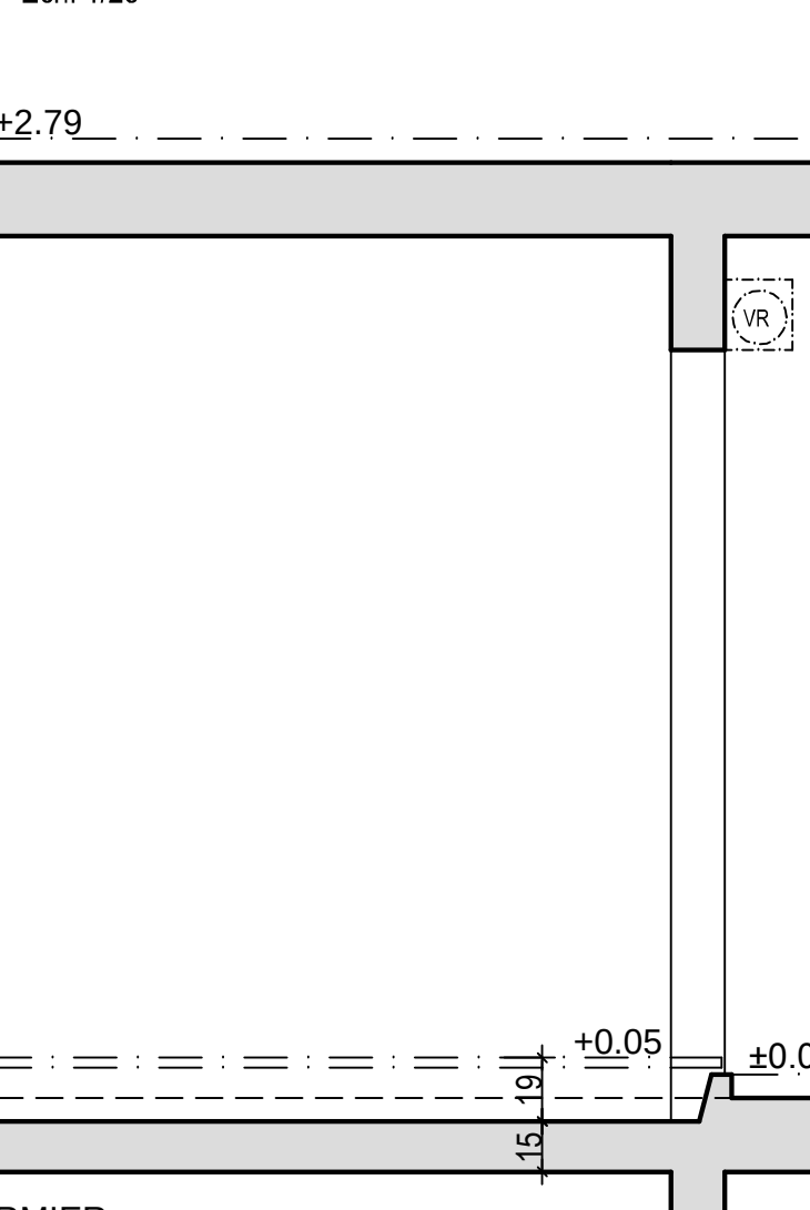
COUPE K Ech: 1/25
