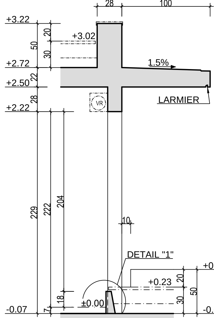
COUPE A Ech: 1/25
