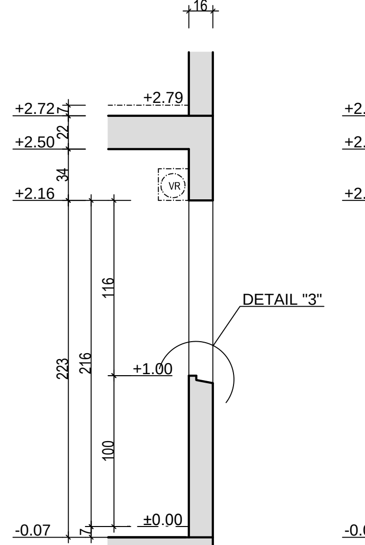
COUPE F Ech: 1/25
