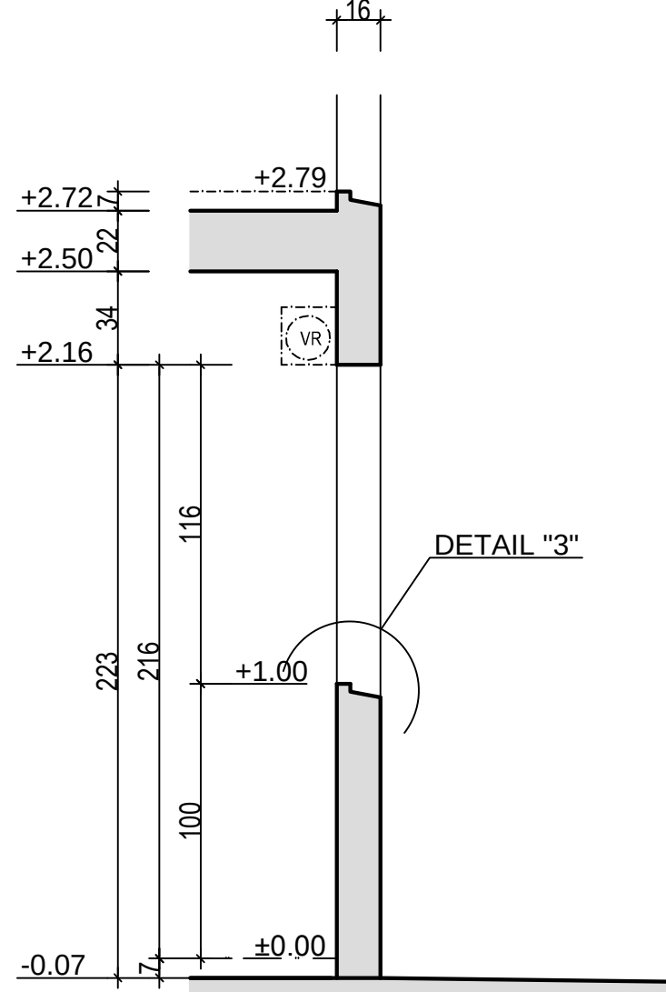
COUPE E Ech: 1/25
