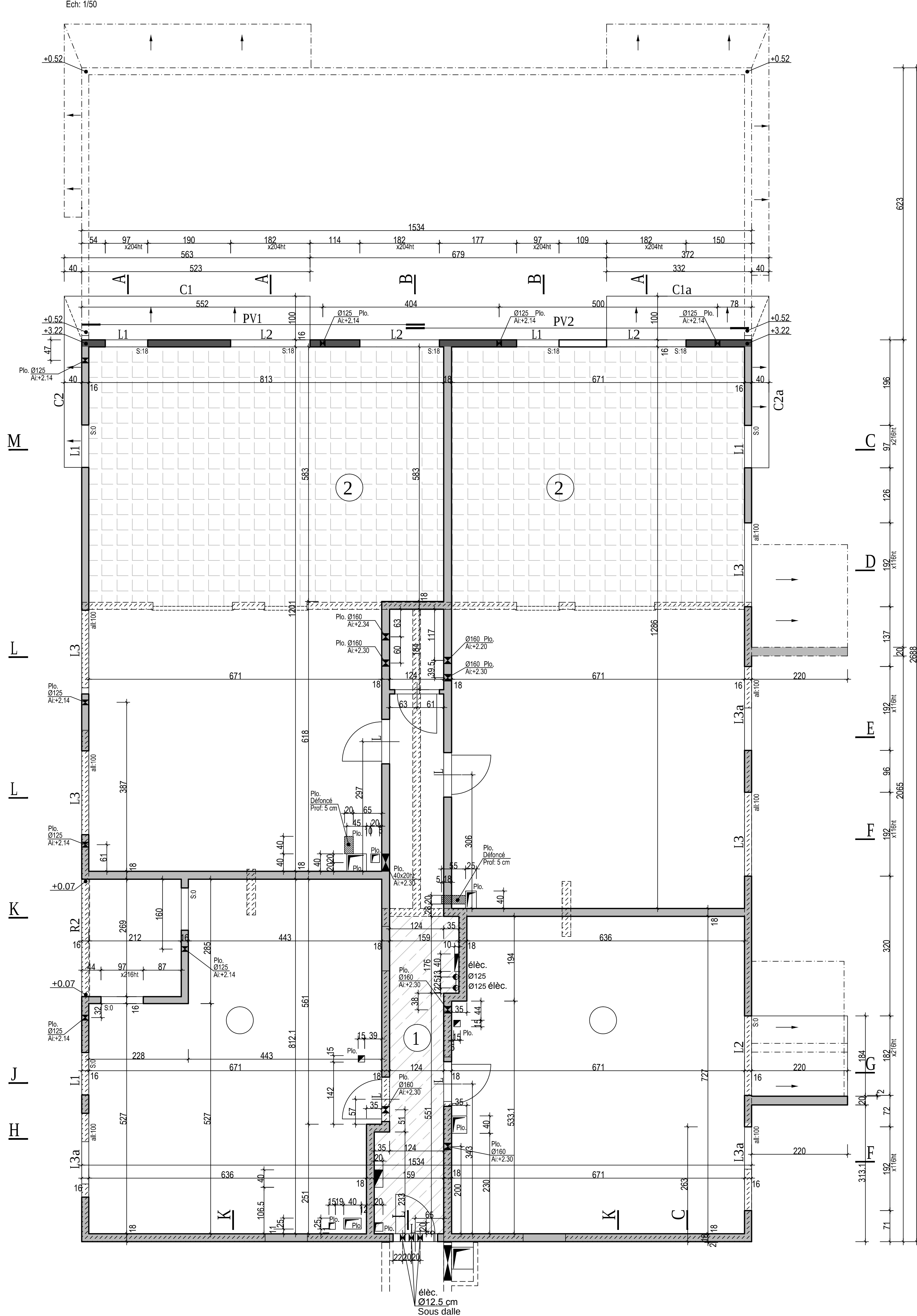
VUE EN PLAN Ech: 1/50
